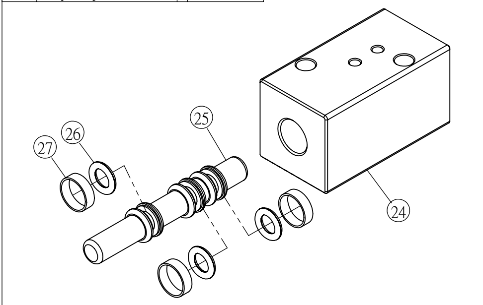
24-27|BodyOfSquareSwitch Set|1|AS451-24-27
